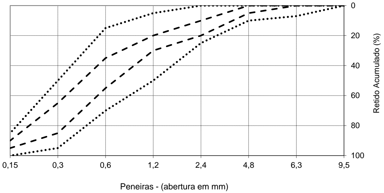
Curva Granulométrica - Agregado Miúdo
