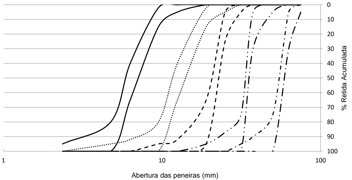
Curva Granulométrica - Agregado Graúdo
