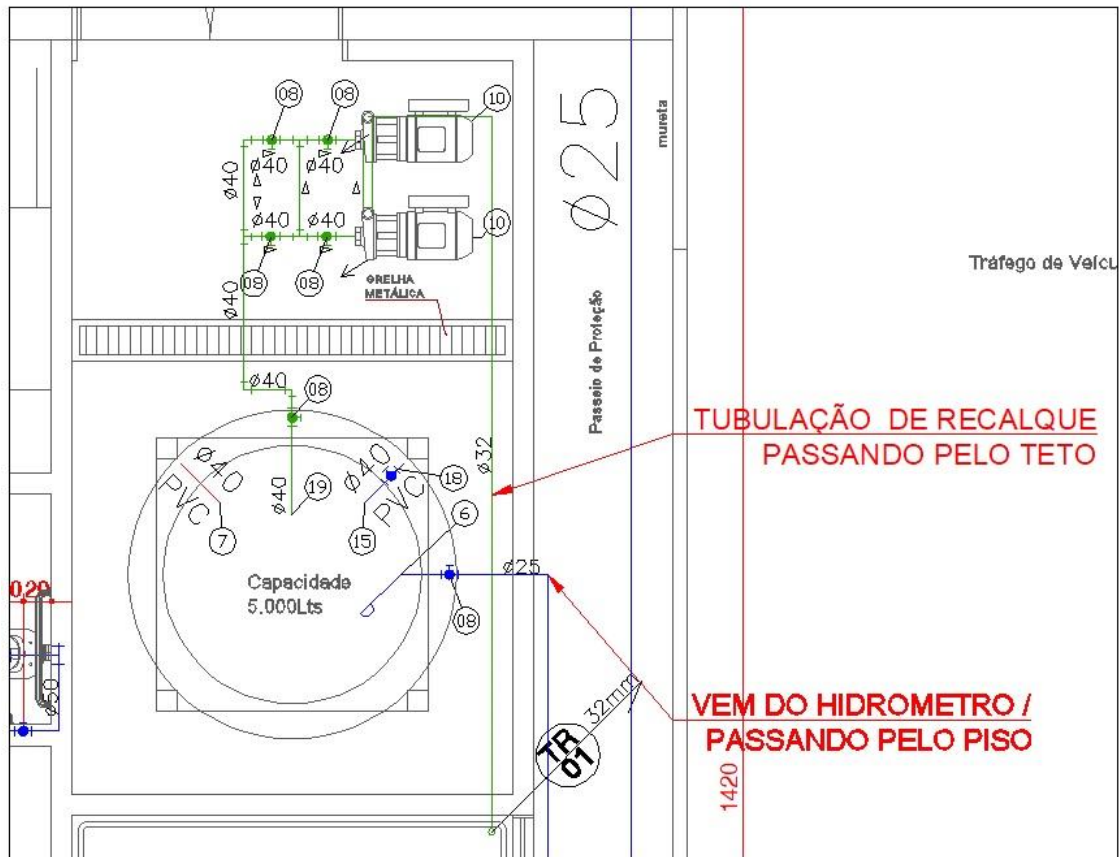
1 PLANTA DO RESERVATÓRIO INFERIOR ESCALA 1:20
