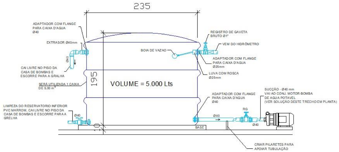
4 CORTE ESQUEMATICO DO RESERVATÓRIO INFERIOR ESCALA 1:20
